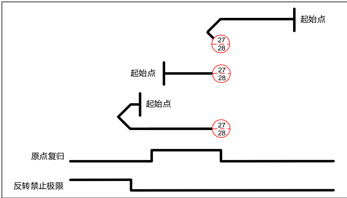
方法 29 及 30：遇反转极限开关和原点开关上缘
