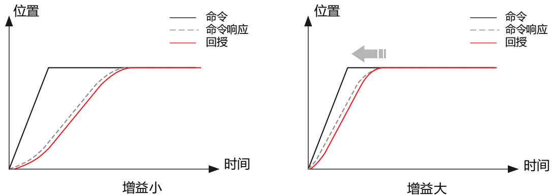
图 5.3.6.1 调整命令带宽响应增益
