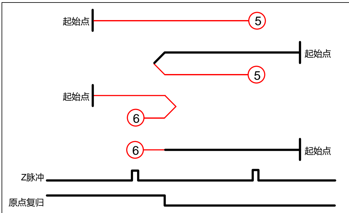
方法 5 及 6: 遇原点开关及参考 Z 脉冲进行复归
