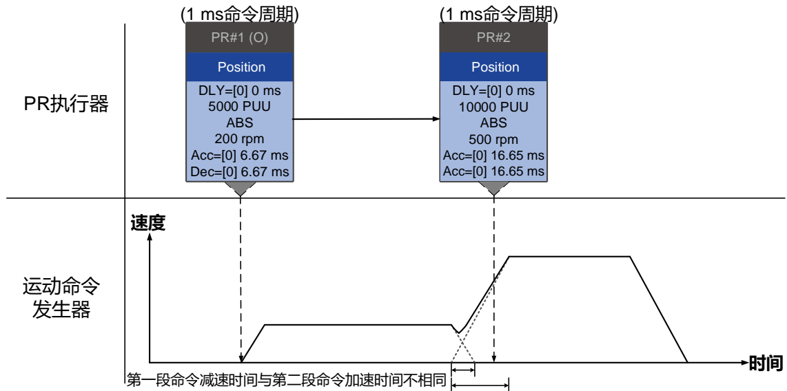
(a) 重送命令 - 加减速时间不同
