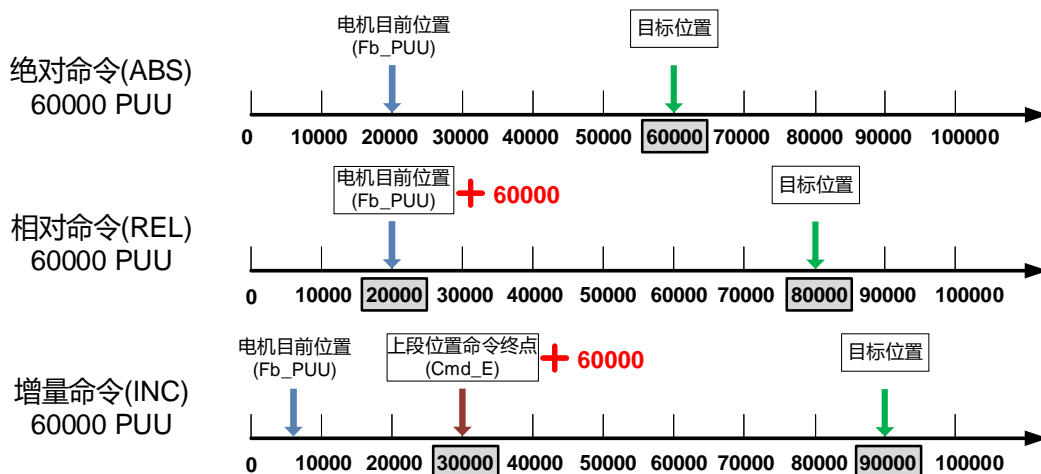
图 7.1.3.3.3 三种位置命令示意图
