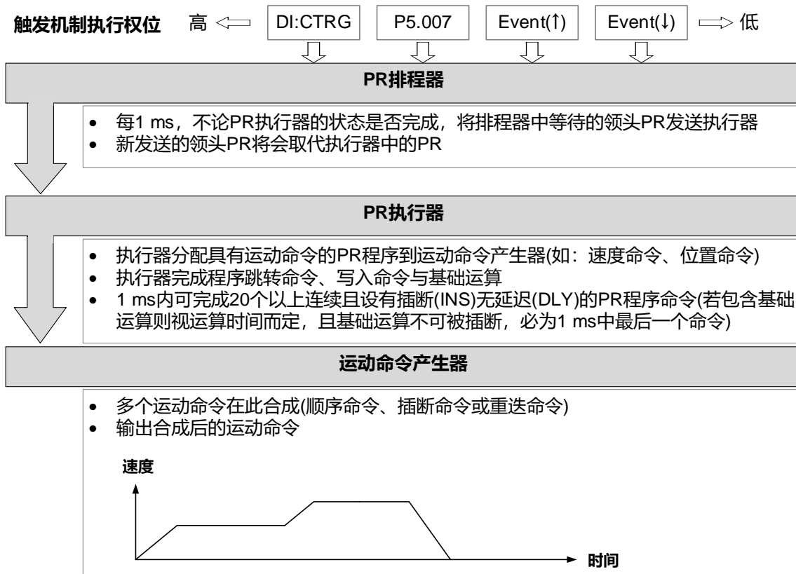
图 7.1.6.1 ASDA-E3 内部 PR 分配机制
