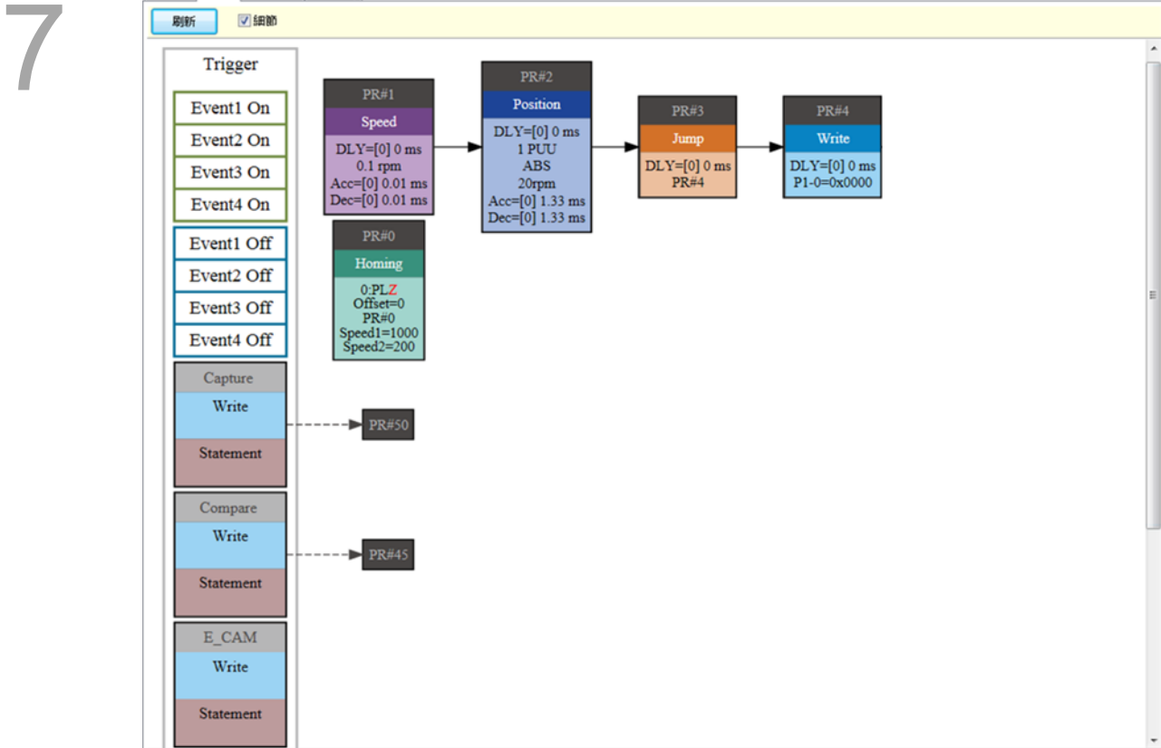
图 7.1.3 ASDA-Soft PR 图形化程序接口
