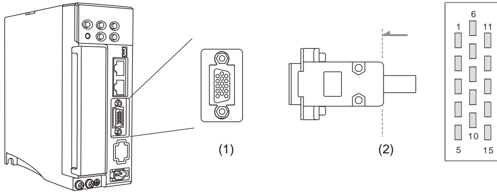
(1) CN1 端子座图；(2) CN1 线端插头配线定义图
