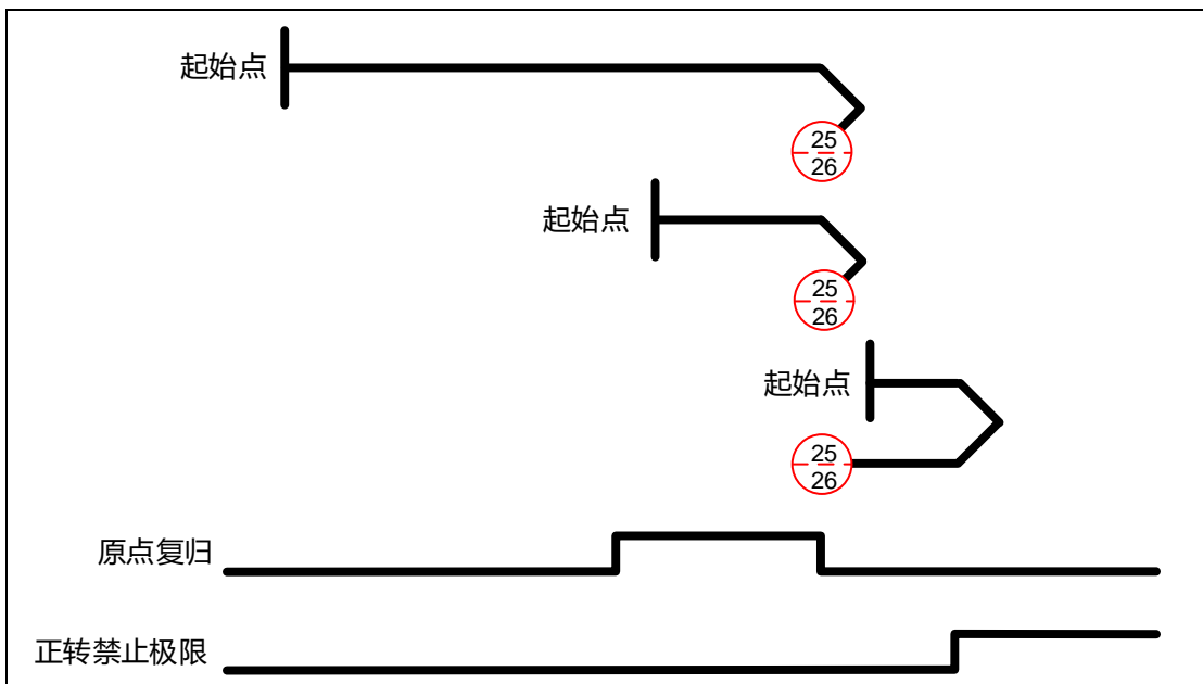
方法 25 及 26: 遇正转极限开关和原点开关
