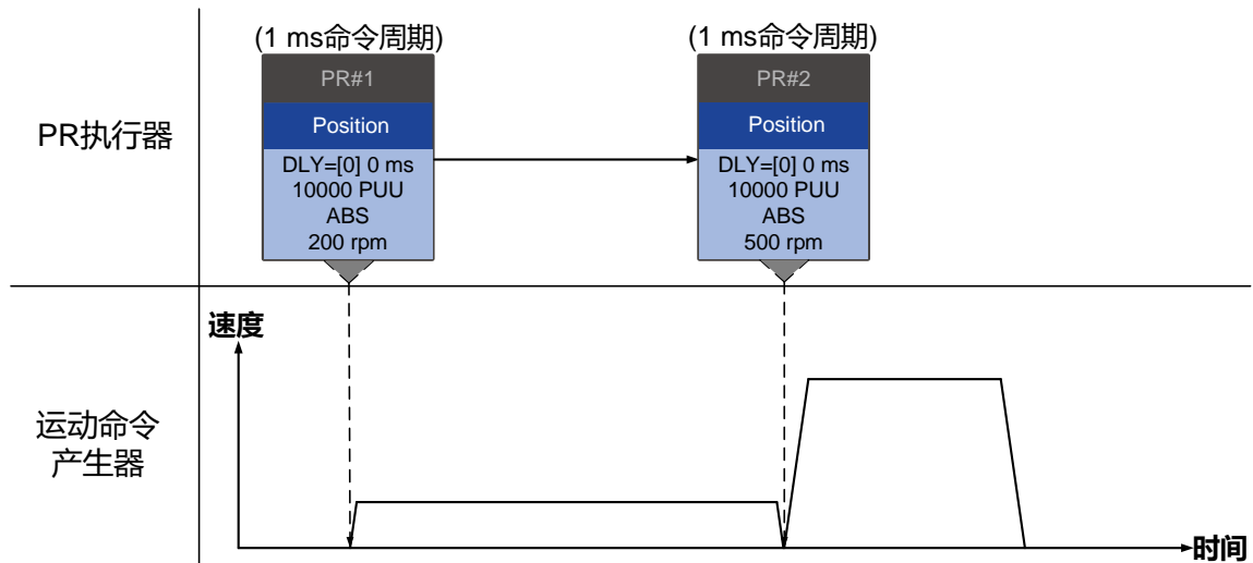
(a) 位置命令无延迟
