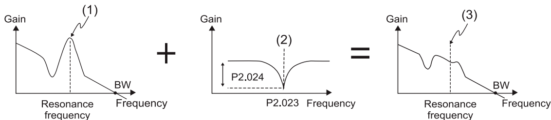
(1) 共振点; (2) 带拒滤波器; (3) 被抑制的共振点
