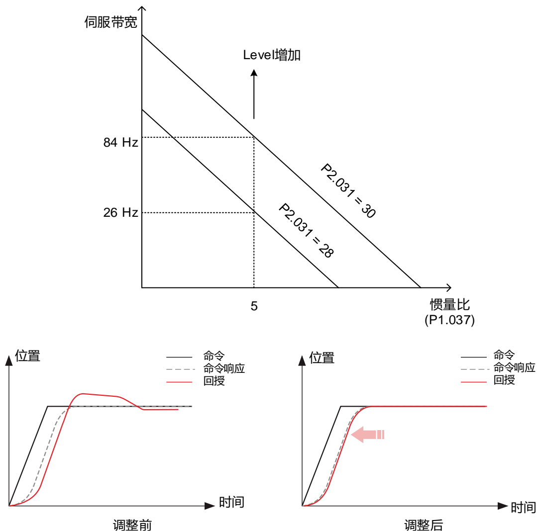
图 5.3.5.1 调整命令带宽响应层级
