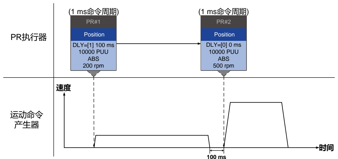
(b) 位置命令有延迟
