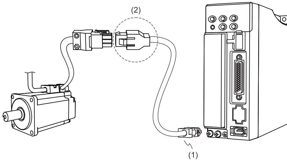
(1) CN2 连接头；(2) 快速接头 (母)
