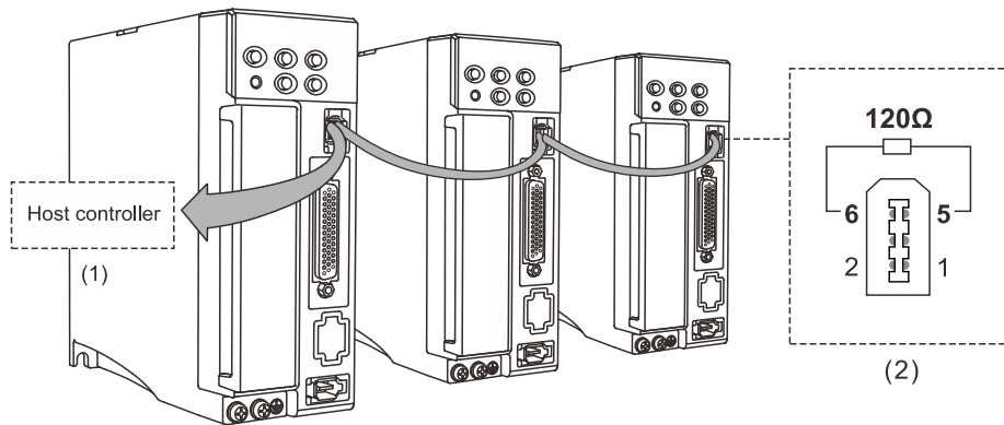
(1) 连接至上位机 / PLC；(2) RS-485 终端电阻接线示意图
