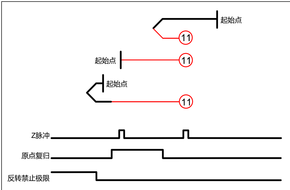
方法 12: 遇反转极限开关, 原点开关和 Z 脉冲进行复归
