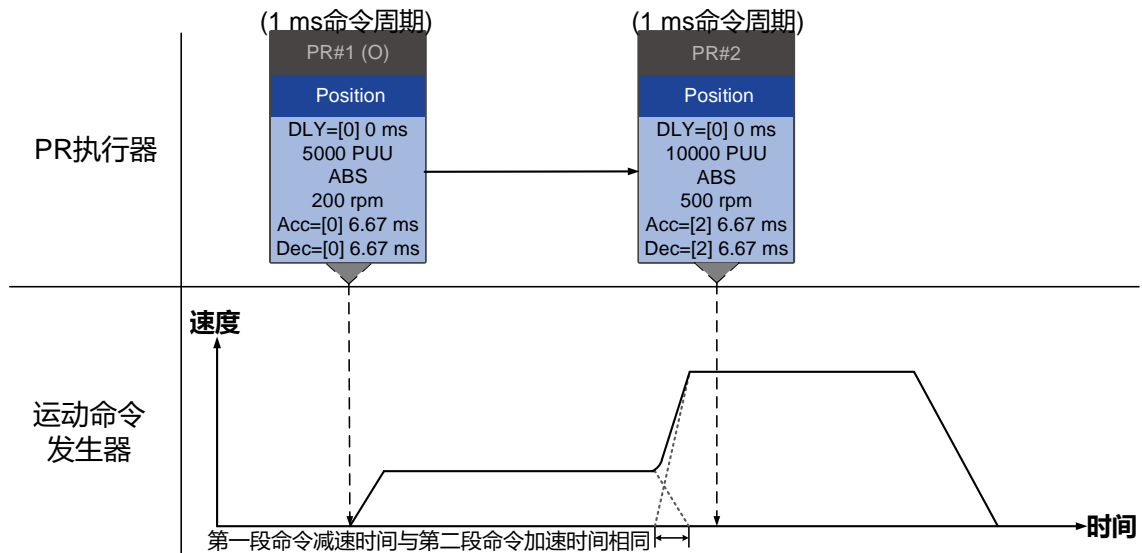
(b) 重送命令 - 加减速时间相同
