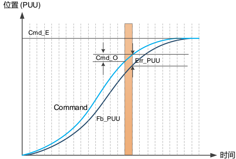
图 7.1.2.2 PR 模式命令执行中监控变量关系示意图
