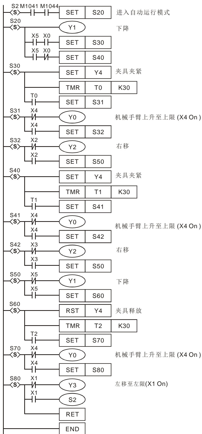
b) 梯形图:
