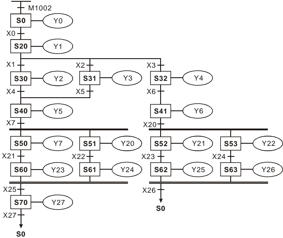
SFC 图:
