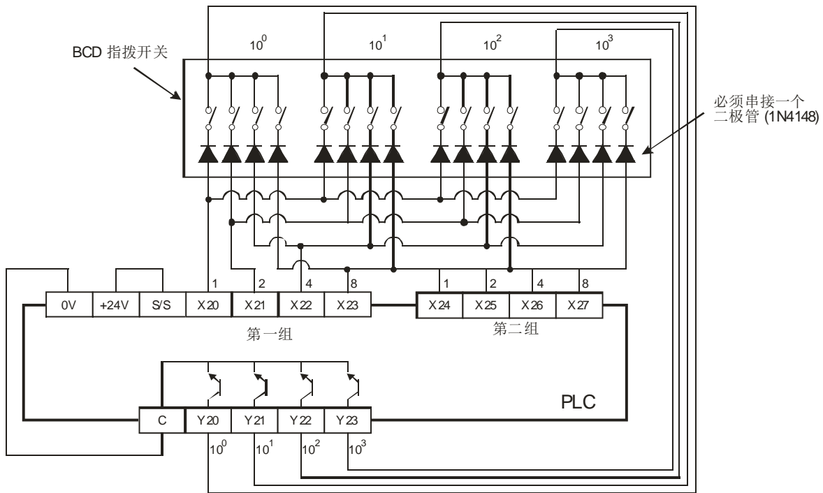
指拨开关输入接线图：
